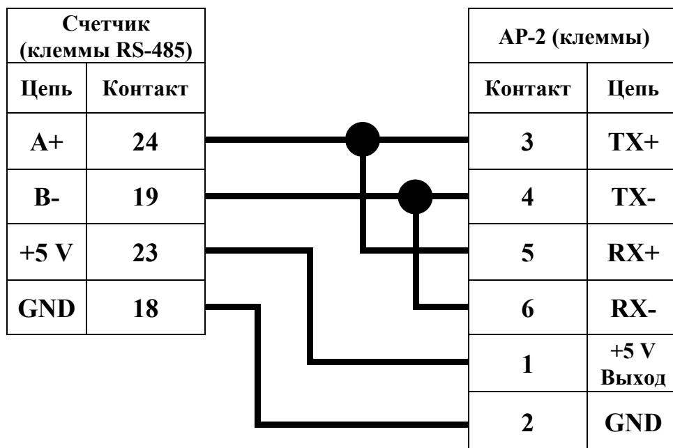
Рисунок А1. Схема соединения AP-2 с Меркурием 230 по интерфейсу RS-485.
