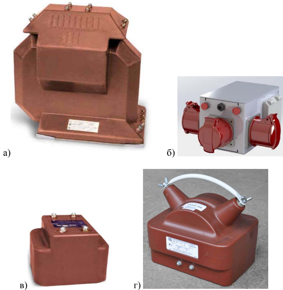
а) – НТ 35 кВ; б) – Коммутатор; в) – НТ 380 В; г) – НТ 10 кВ
