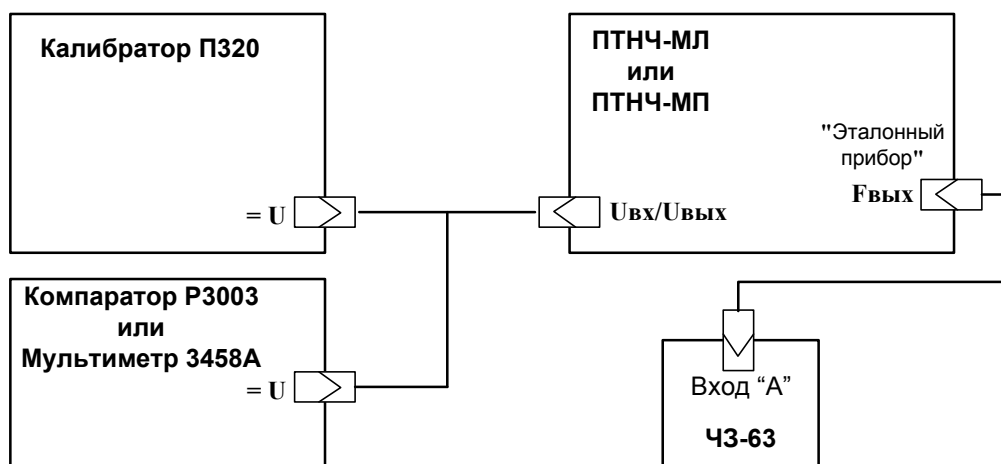
Рисунок А.4. Схемы подключения Приборов модификаций ПТНЧ-МЛ и ПТНЧ-МП для определения основной погрешности измерения напряжения постоянного тока и преобразования его в частоту следования импульсов
