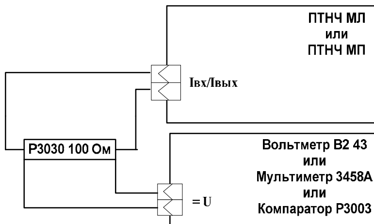
Рисунок А.11. Схема подключения Приборов модификаций ПТНЧ-МЛ и ПТНЧ-МП для определения основной погрешности воспроизведения силы постоянного тока. Значение силы тока в мА численно равно 10 \cdot U , где U - измеренное значение напряжения в Вольтах.
