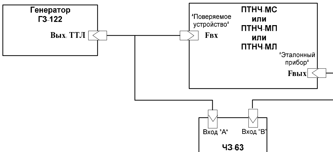
Рисунок А.1. Схема подключения Приборов при проверке работы в режиме деления частоты
