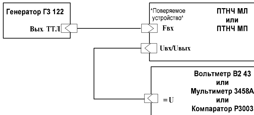
Рисунок А.7. Схема подключения Приборов модификаций ПТНЧ-МЛ и ПТНЧ-МП для определения основной погрешности измерительного преобразования частоты следования импульсов в напряжение постоянного тока
