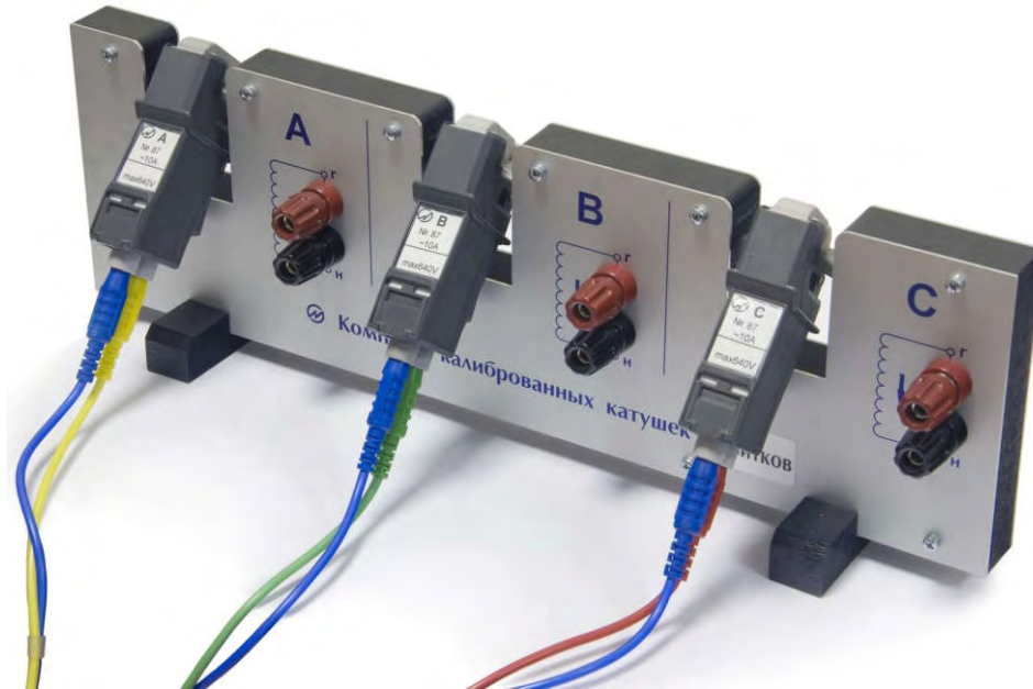
Рисунок 2.4.1 Катушка токовая калиброванная КТ-3-20 (или КТ-3-10)
