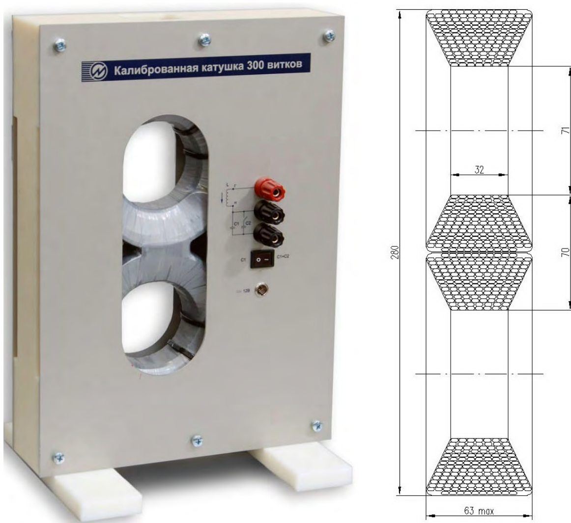
Рисунок 2.4.3 Катушка токовая калиброванная КТ-1-300 (или КТ-1-200)
