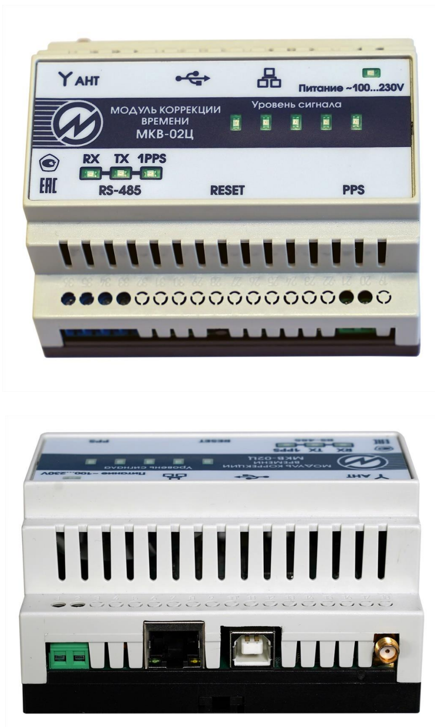
Рис. 3.1. Расположение соединителей, клемм и индикаторов Модуля МКВ-02Ц
