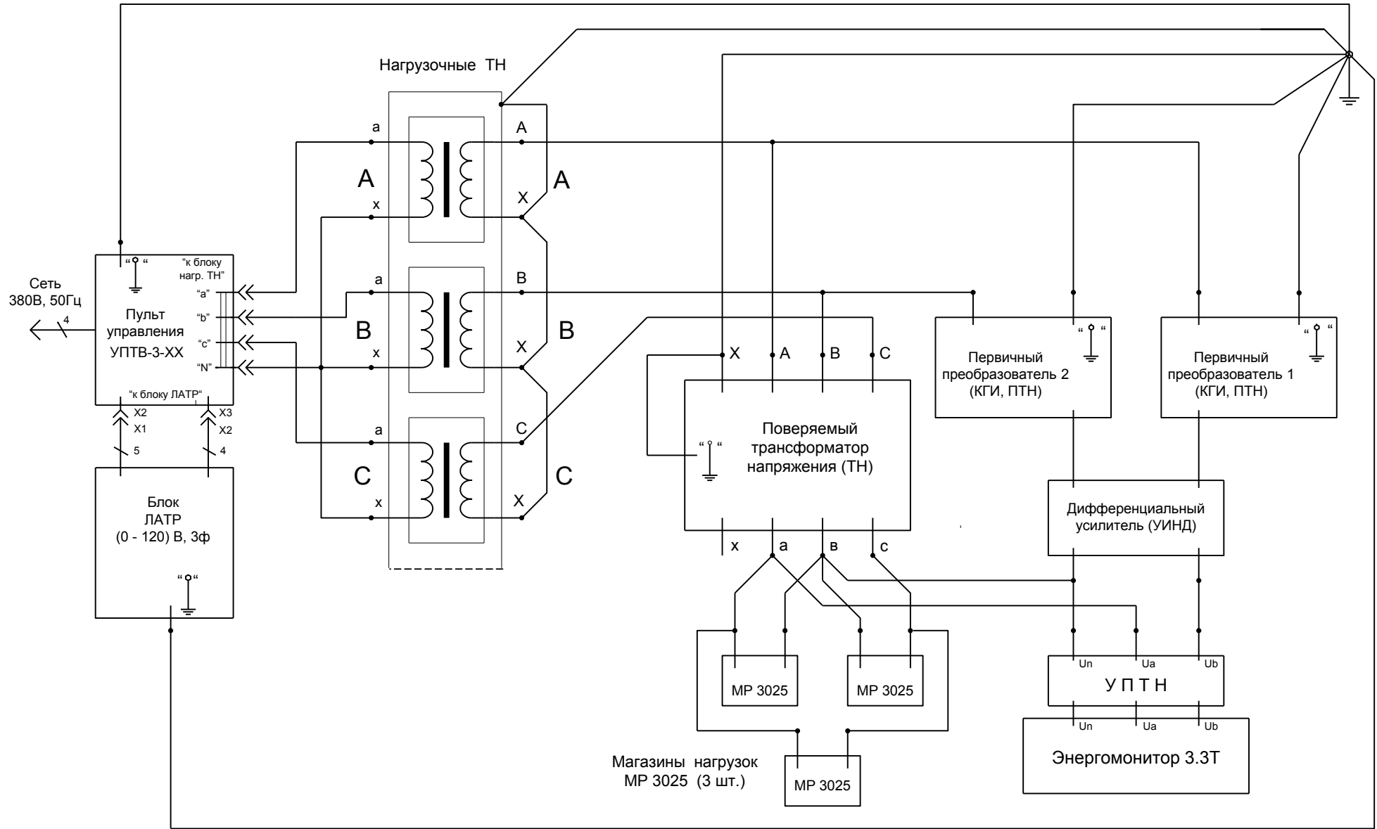
Схема 2 поверки ТН (2 ПВЕ, «треугольник»)
