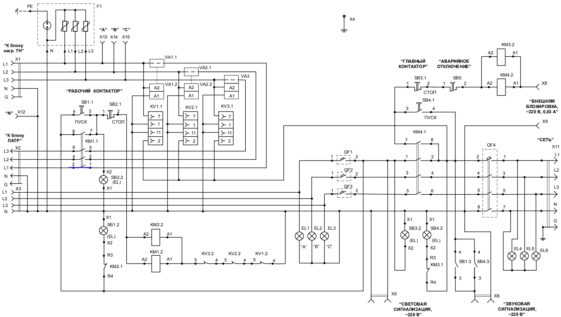
Рис. 2. Схема электрическая ПУ УПТВ-3-XX
