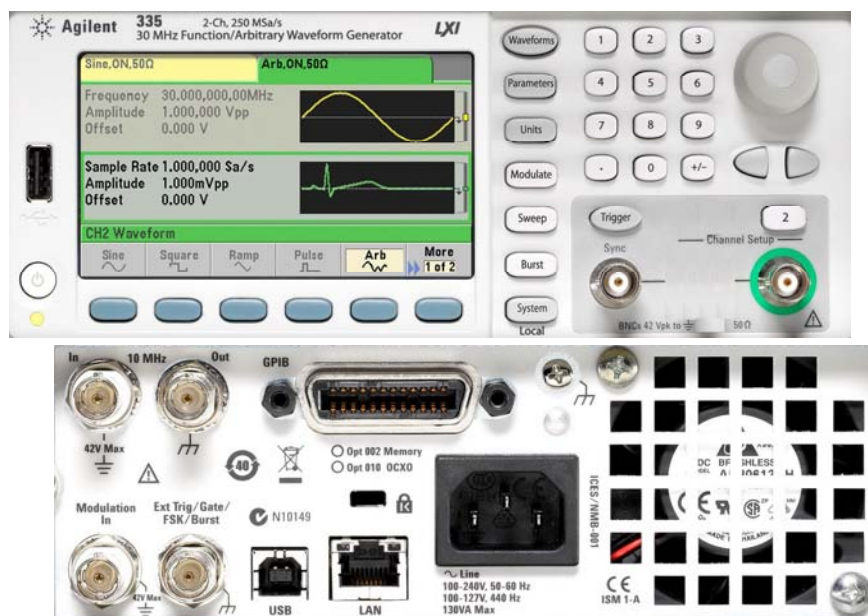
Рисунок 2.4 - Генератор сигналов произвольной формы "33521В"
