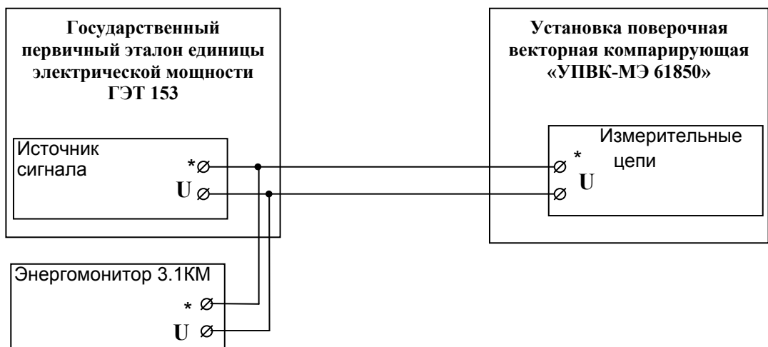
Рисунок А.4 Схема подключения УПКВ при определении погрешности измерения суммарного коэффициента гармонических составляющих напряжения
