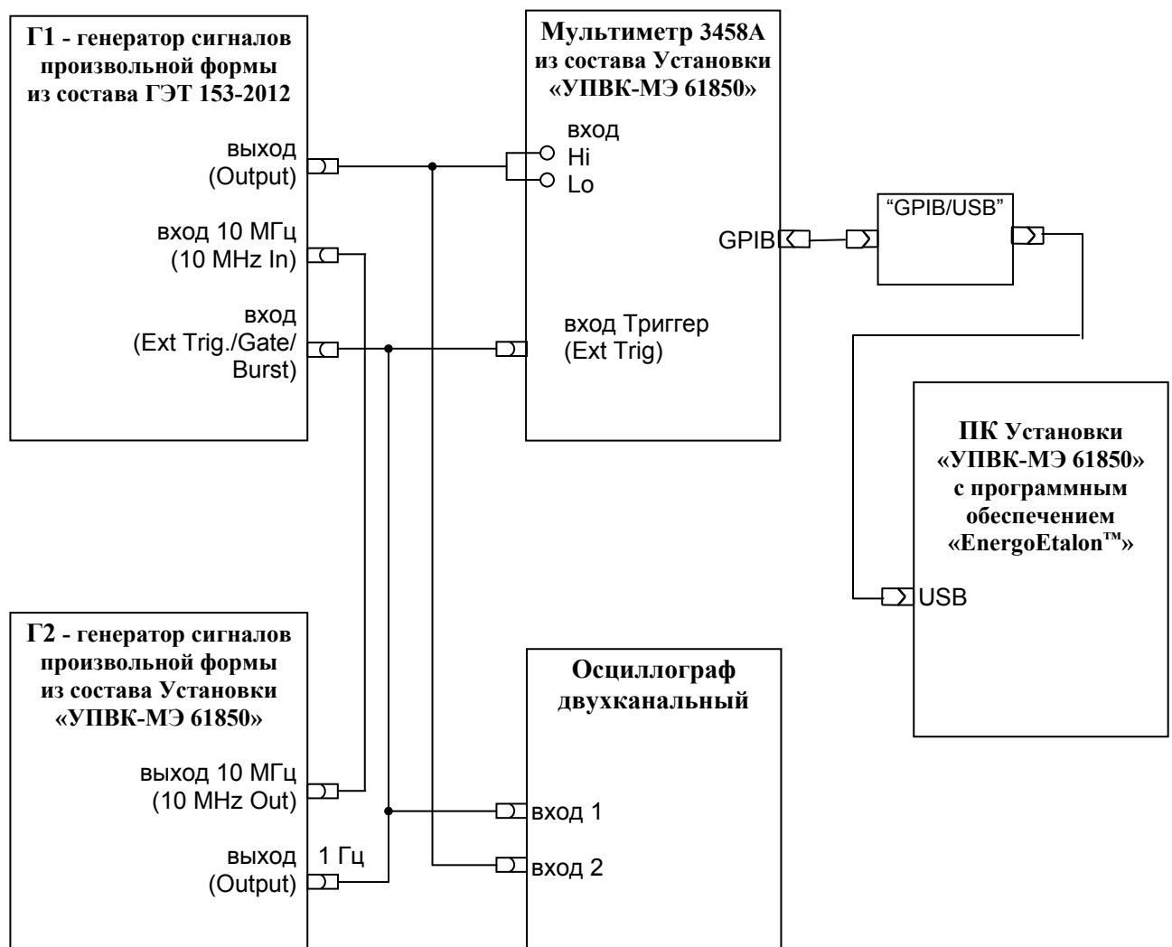
Рисунок А.6 Схема подключения УПВК при определении абсолютной погрешности угла сдвига фаз между основной гармоникой напряжения и опорным сигналом 1 Гц (PPS)
