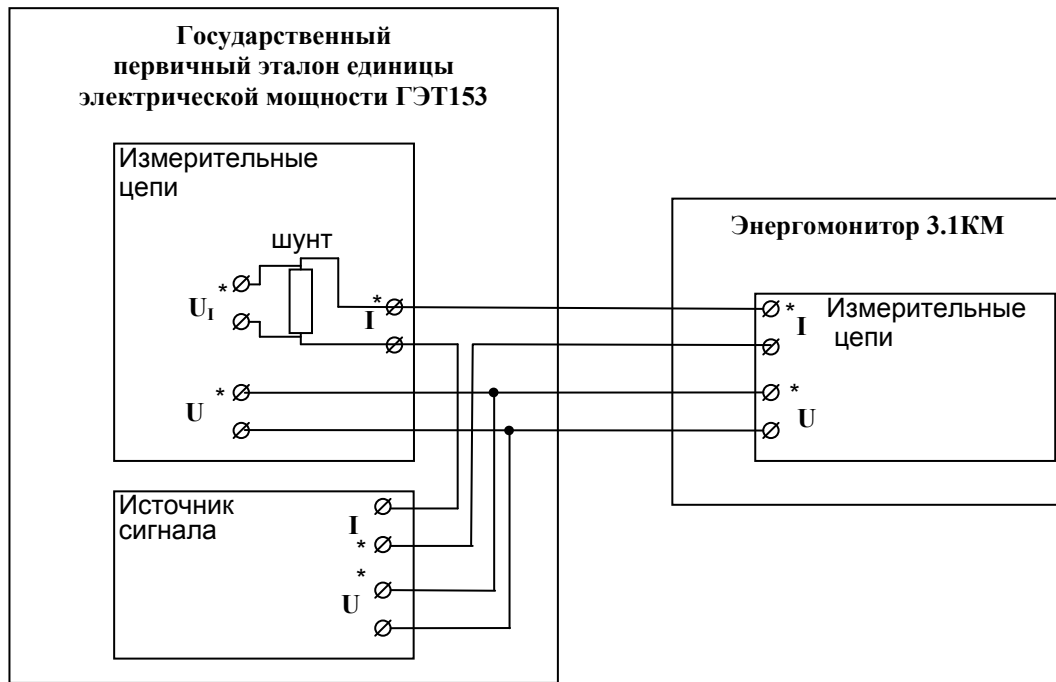
Рисунок А.7 Схема подключения УПКВ при определении абсолютной погрешности угла сдвига фаз между током поданным на шунт и напряжением на выходе шунта
