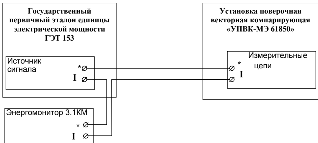
Рисунок А.5 Схема подключения УПВК при определении погрешности измерения суммарного коэффициента гармонических составляющих тока
