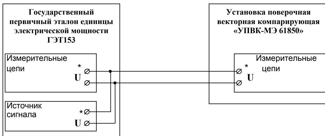
Рисунок А.1. Схема подключения УПК к ГЭТ153-2012 при измерении напряжения.
