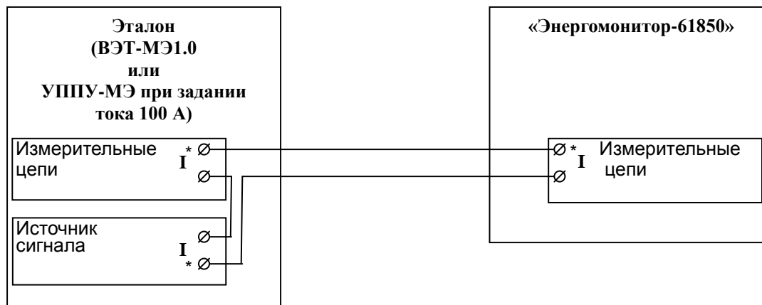
Рисунок А.2 - Схема подключения прибора Энергомодитор-61850 к эталону при измерении тока.
