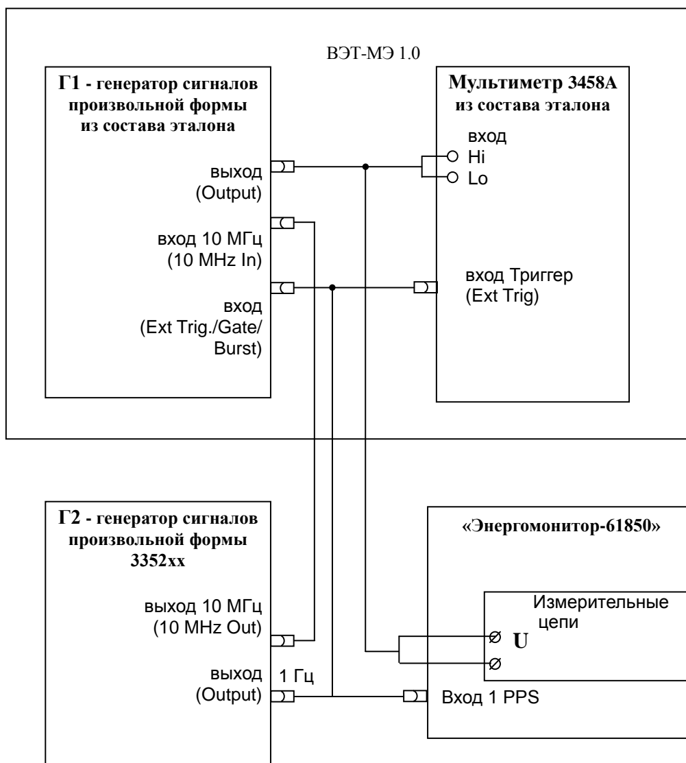
Рисунок А.5 - Схема подключения прибора Энергомонитор-61850 при определении абсолютной погрешности угла сдвига фаз между основной гармоникой напряжения и опорным сигналом 1 Гц (PPS)
