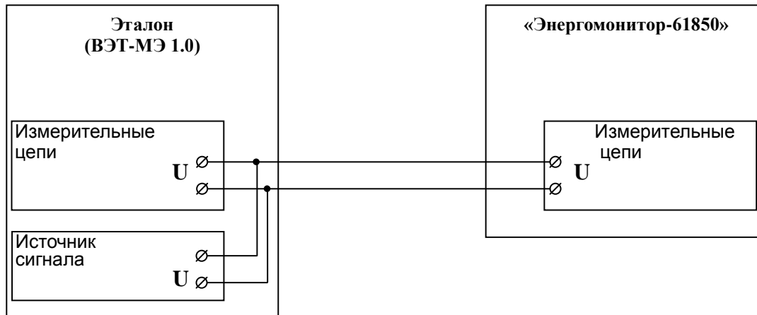
Рисунок А.1 - Схема подключения прибора Энергомодитор-61850 к эталону при измерении напряжения.
