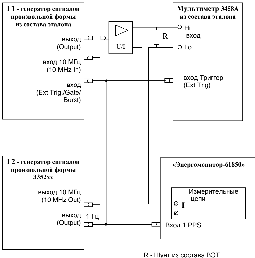
Рисунок А.6 - Схема подключения прибора Энергомонитор-61850 при определении погрешности определения угла сдвига фазы между основной гармоникой тока и опорным сигналом 1 Гц (PPS)
