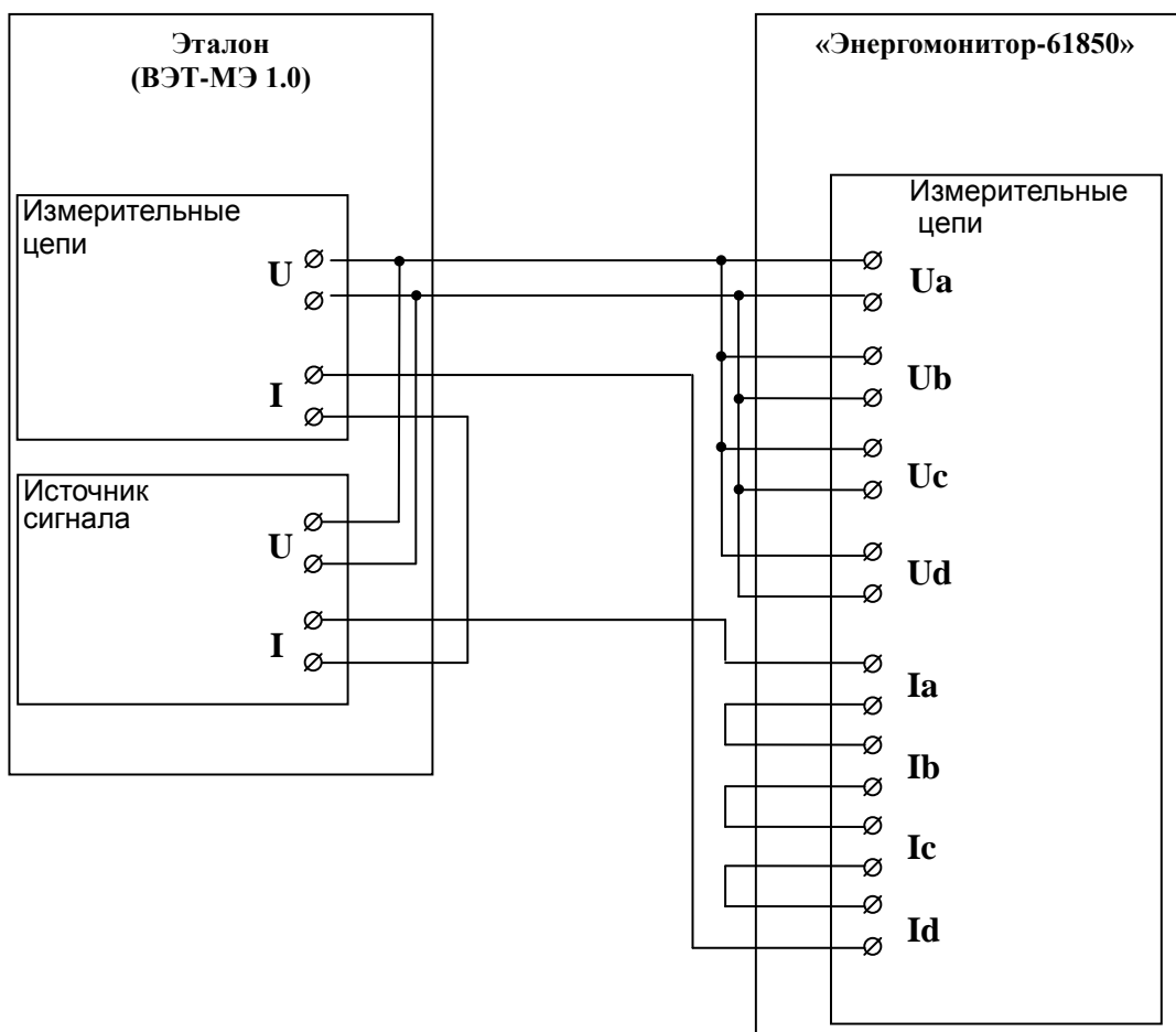
Рисунок А.3 - Схема подключения прибора Энергомонитор-61850 при измерении электрической мощности и при определении погрешности измерения суммарного коэффициента гармонических составляющих тока.
