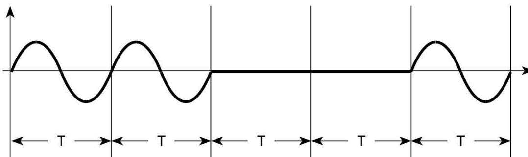
Рис. 4.15. Форма выходного сигнала в режиме «Субгармоники» ( T — период сигнала)
