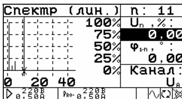
Рис. 4.11. Окно «Форма сигнала» в варианте представления «Спектр (линейный)»
