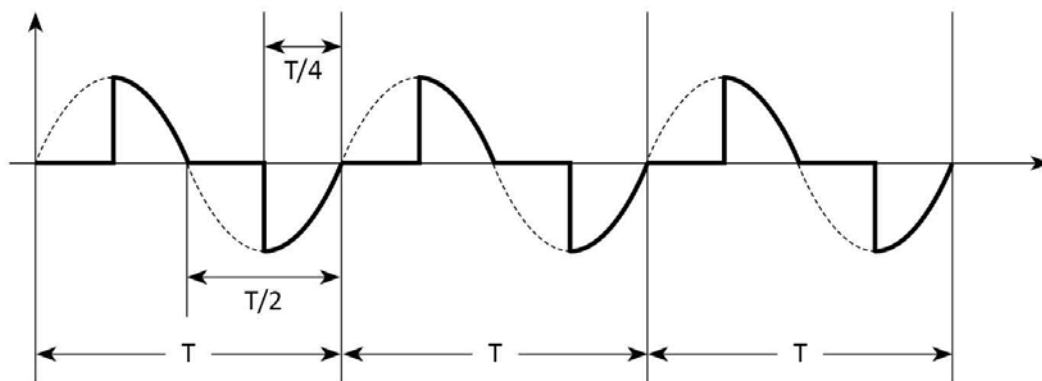
Рис. 4.17. Форма выходного сигнала в режиме «Фазовое управление» (T — период сигнала)
