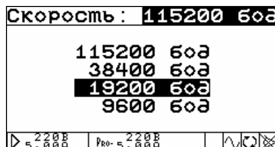
Рис. 4.22. Меню выбора скорости обмена с ПК по интерфейсу RS-232
