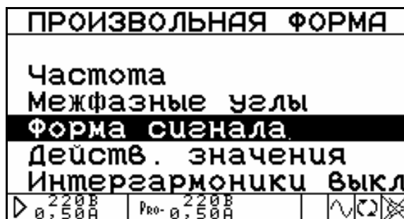
Рис. 4.7. Меню «Произвольная форма»
