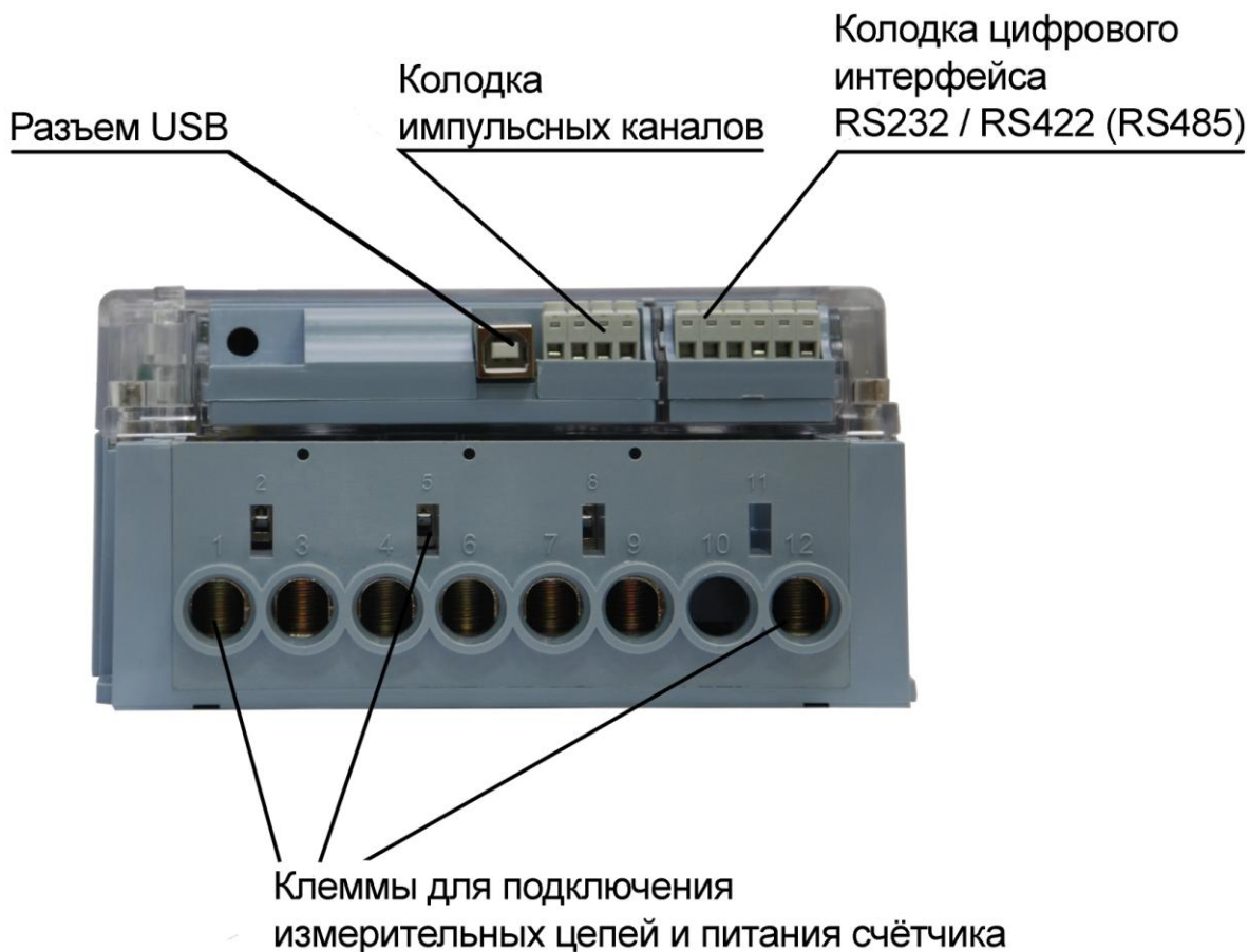
Рисунок 7.1.2 – Расположение клемм и интерфейсов счетчика СКВТ-Φ-МАРСЕН.
