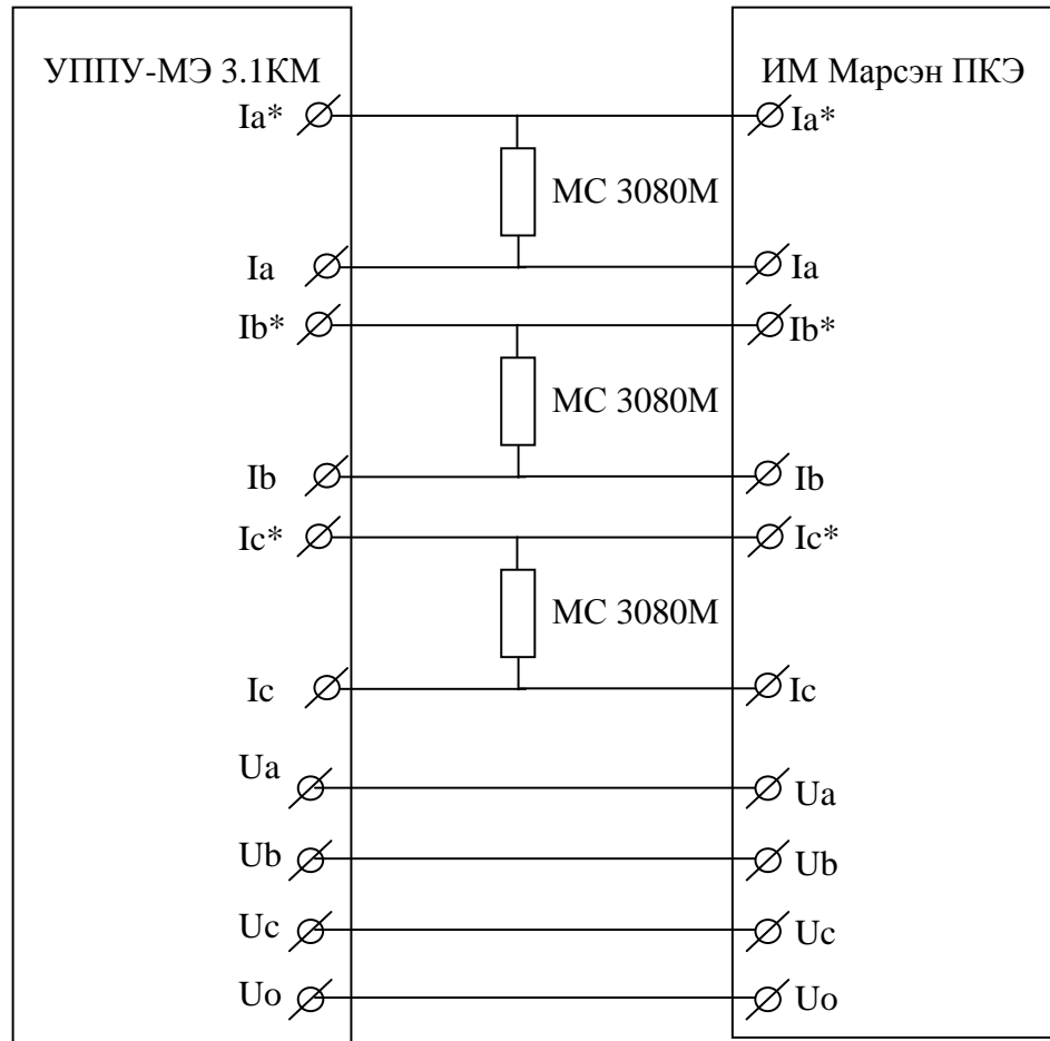
Рисунок А2 - Трехфазная четырехпроводная схема подключения «ИП Марсен-ПКЭ-vvvv» к УППУ-МЭ 3.1КМ (ток 1 А)
