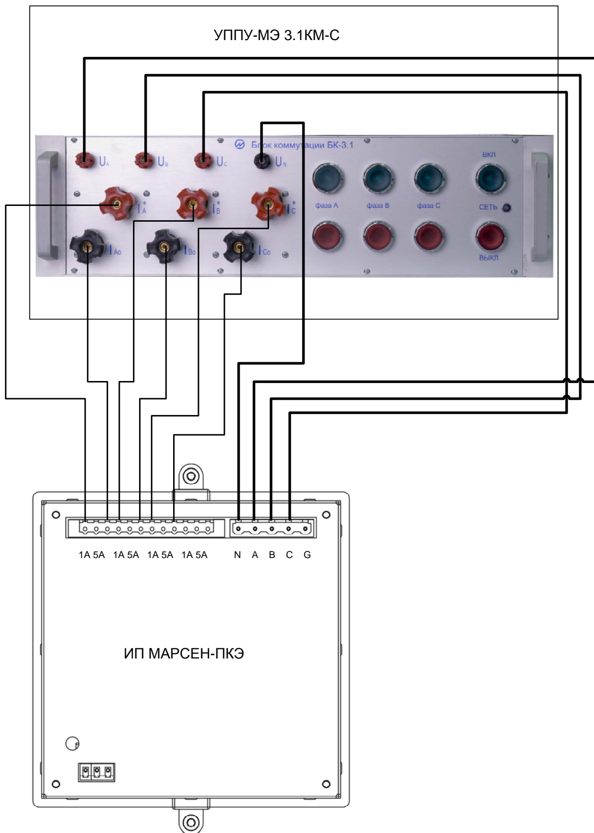
Рисунок А.1 - Трехфазная четырехпроводная схема подключения «ИП Марсен-ПКЭ-1/5» к УППУ-МЭ 3.1КМ (ток 1 А)
