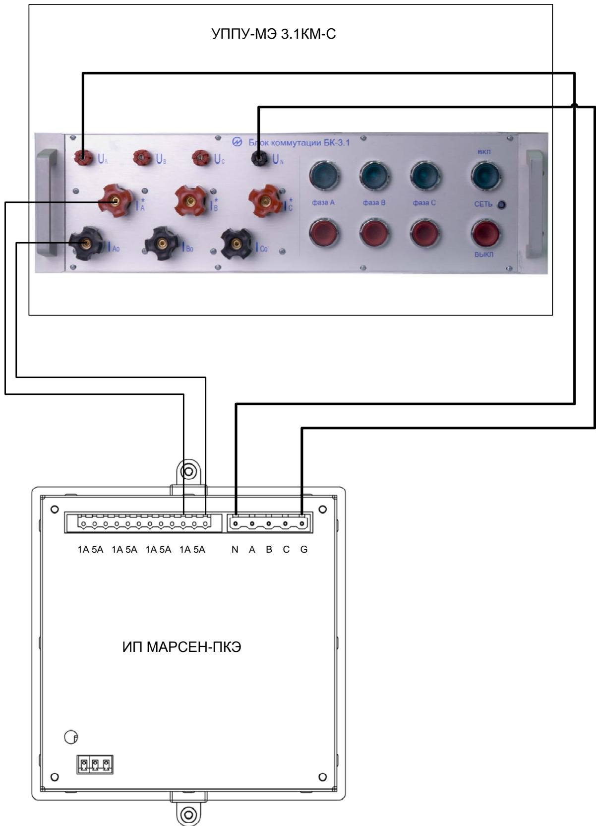
Рисунок А.3 - Схема подключения входов нейтрали «ИП Марсен-ПКЭ 1/5» к УППУ-МЭ 3.1КМ (ток 1 А)
